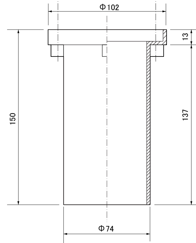
【土台部正面図】
